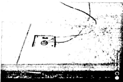
लेबर रूम में अव्यवस्थित विद्युत वायरिंग
